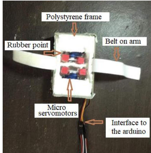
Fig. 13. Actuator system
